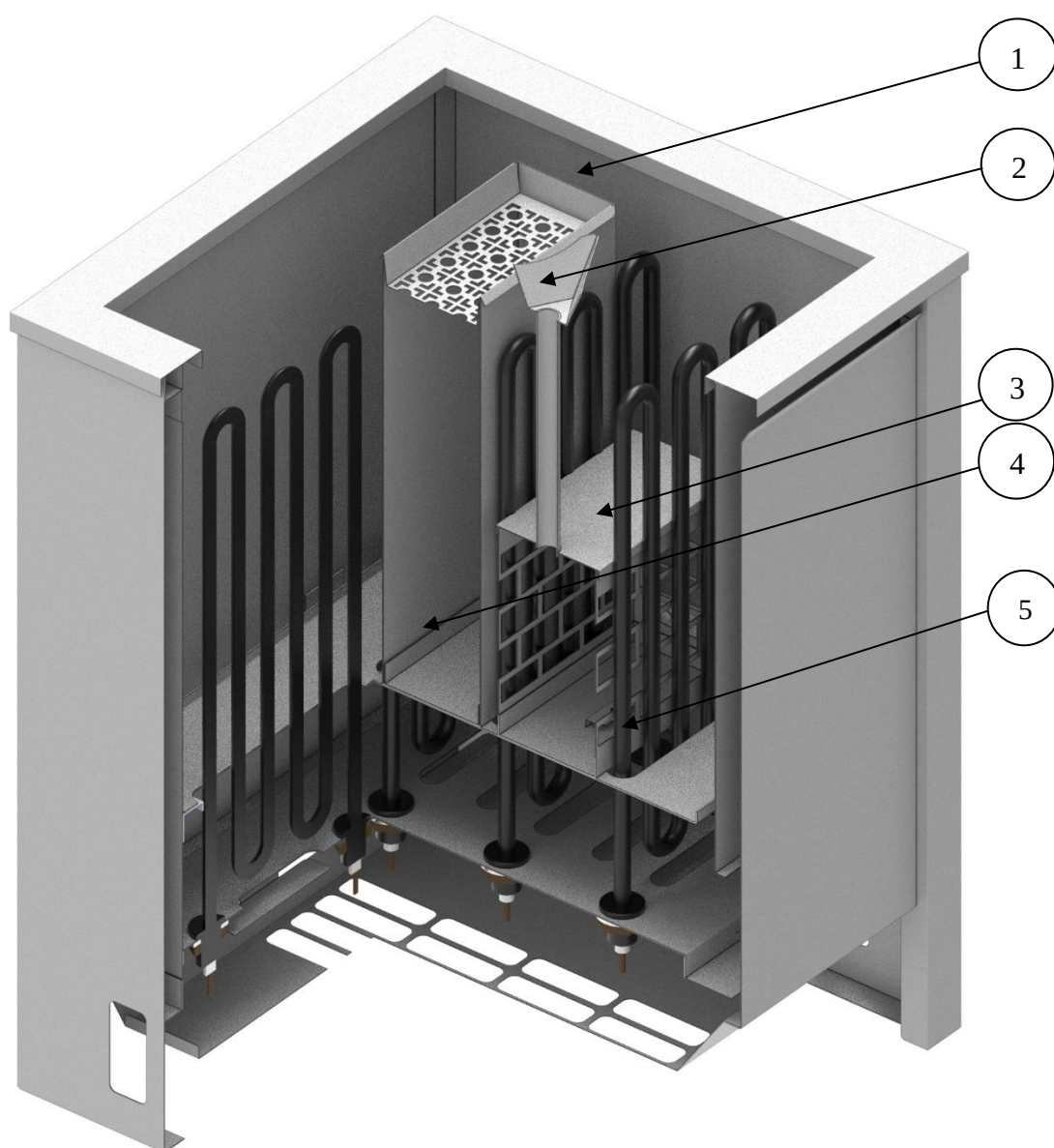
Рис. 5. Взаимное расположение составных частей изделия CLASSIC: 1- Корпус, 2 - Воронка для долива воды в корзину для камней, 3 – Корзина для камней, 4 – Бак для воды, 5- Бак для воды, 6 – ТЭНы.
