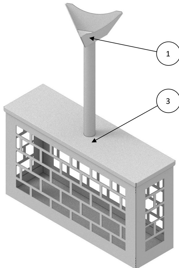
Рис. 9. Сетка для камней. Изометрическая проекция.
