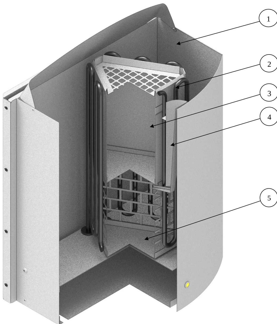
Рис. 3. Взаимное расположение составных частей изделия OPTIMA STEAM: 1- Корпус наружный, 2 – ТЭНы, 3 – Бак для воды с сеткой, 4 – Воронка для долива воды, 5- Сетка для камней.
